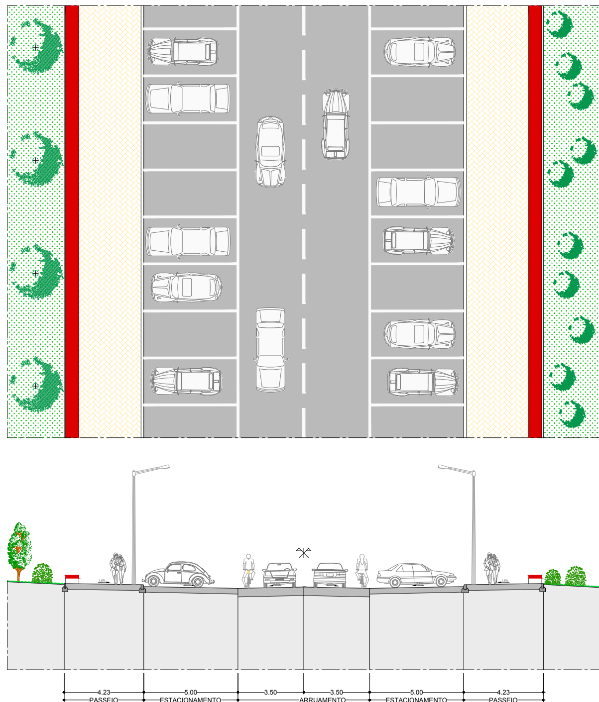
PERFIL TRANSVERSAL PT 6
