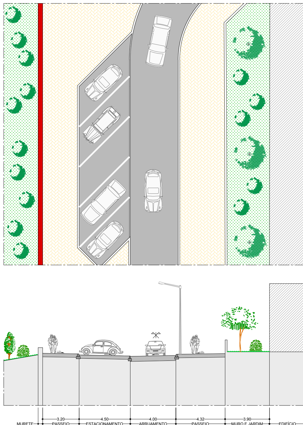
PERFIL TRANSVERSAL PT 7
