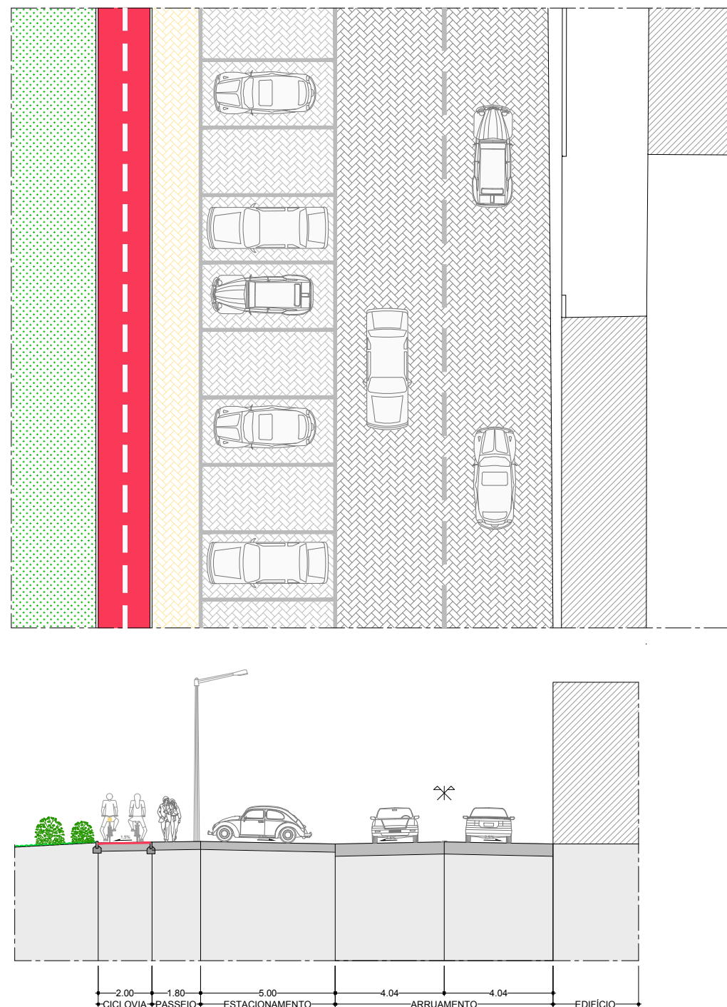
PERFIL TRANSVERSAL PT 4
