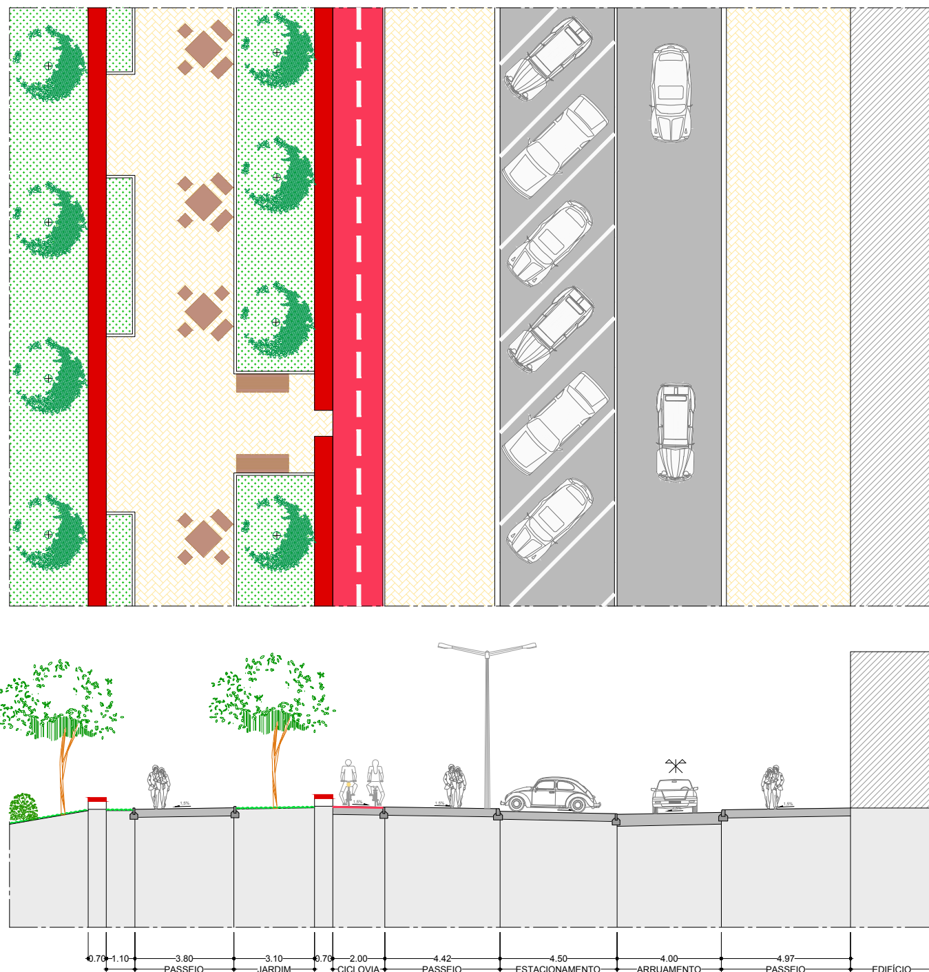
PERFIL TRANSVERSAL PT 5
