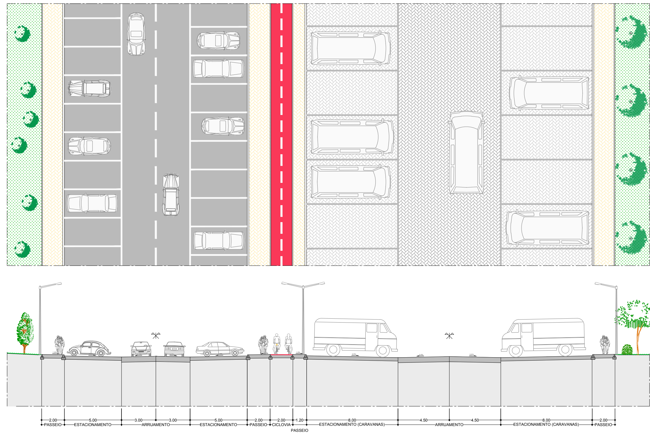
PERFIL TRANSVERSAL PT 1
