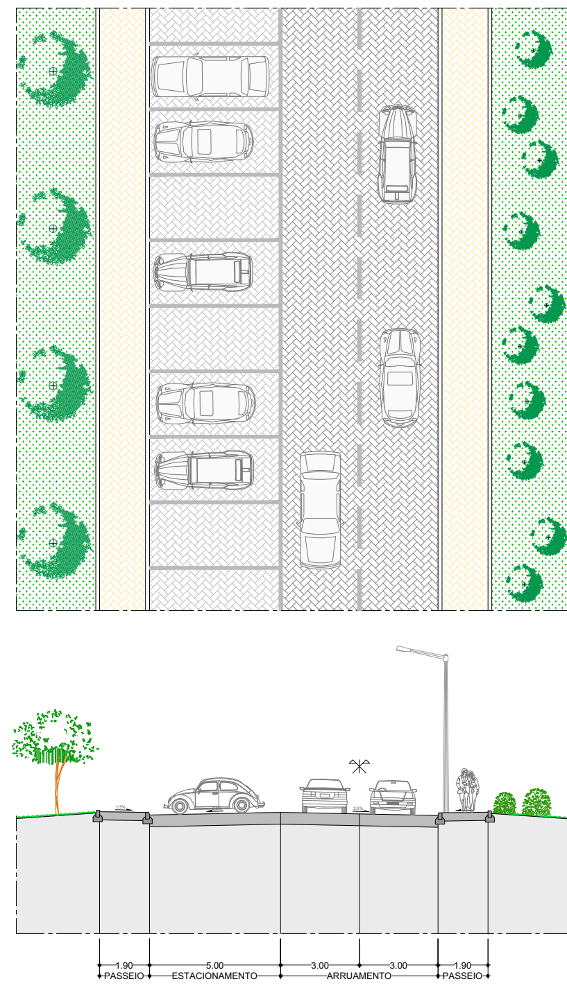
PERFIL TRANSVERSAL PT 3
