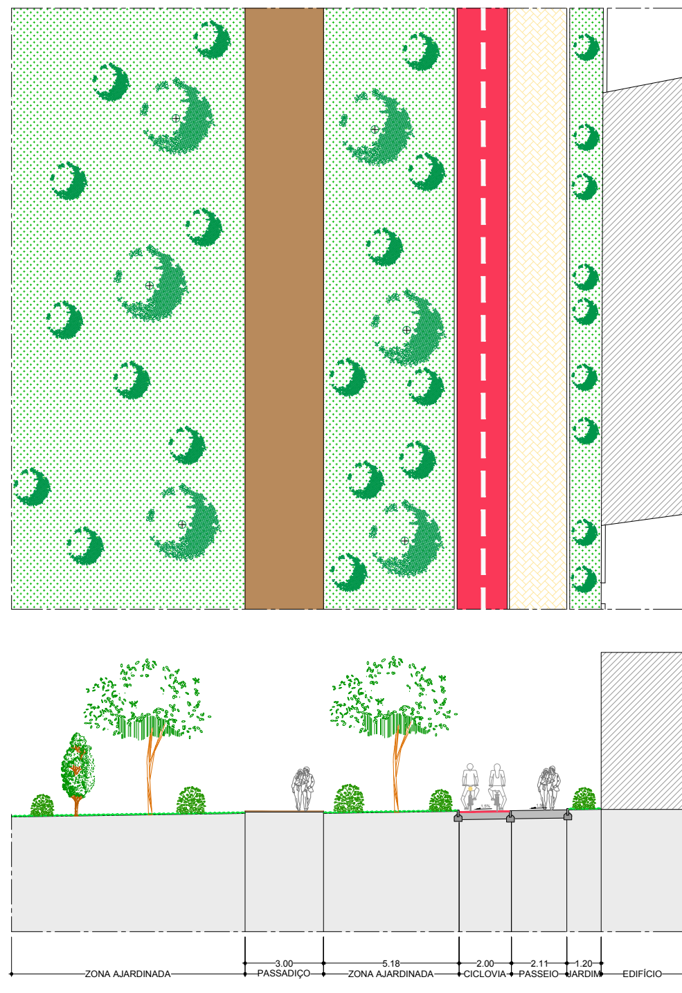
PERFIL TRANSVERSAL PT 2
